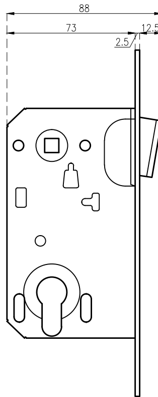
widok z boku (element 1)
